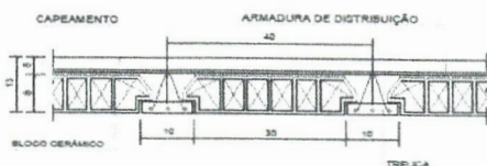
DETALHE LAJE TRELIÇADA SIMPLES
